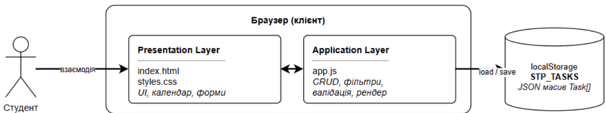
Рисунок 1 – діаграма архітектури
