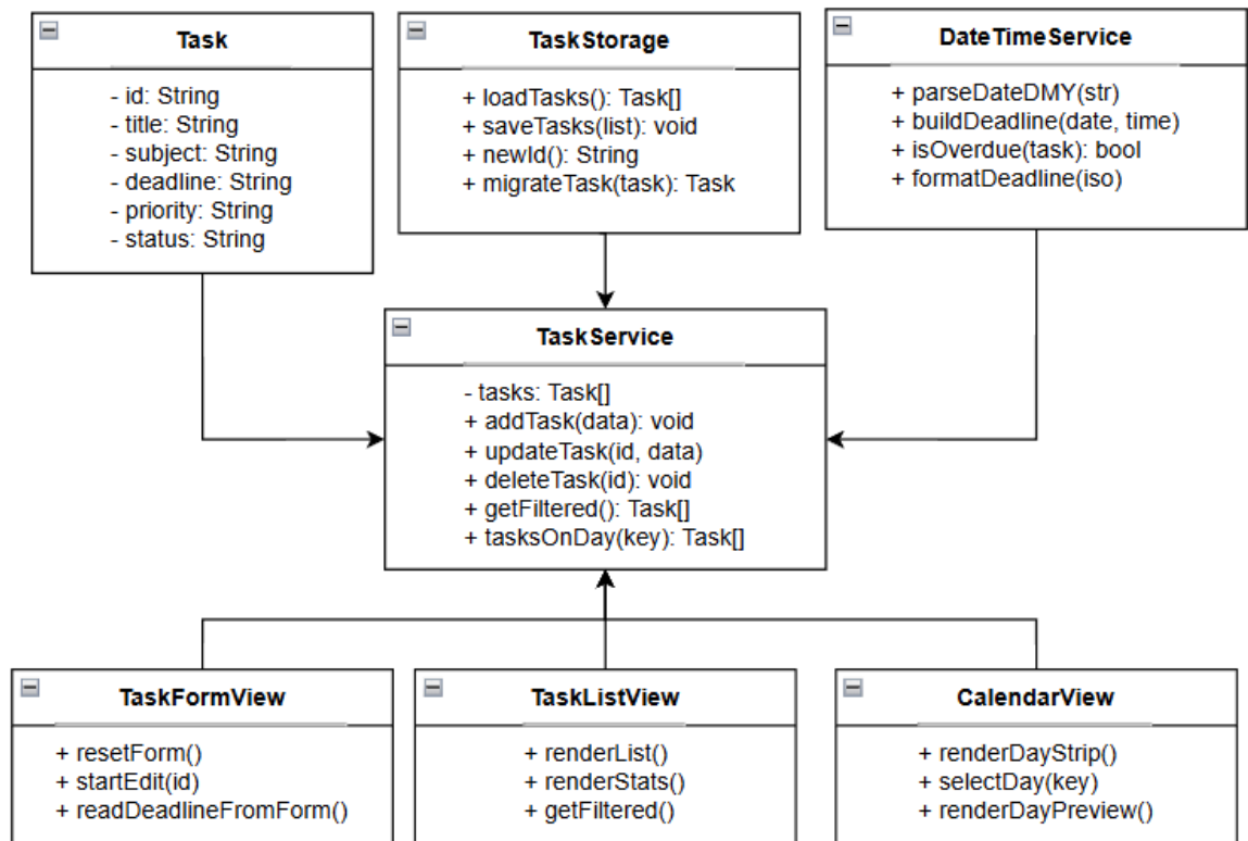
Рисунок 2 – діаграма класів
