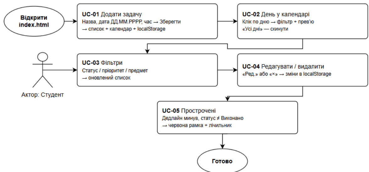
Рисунок 3 – діаграма сценаріїв
